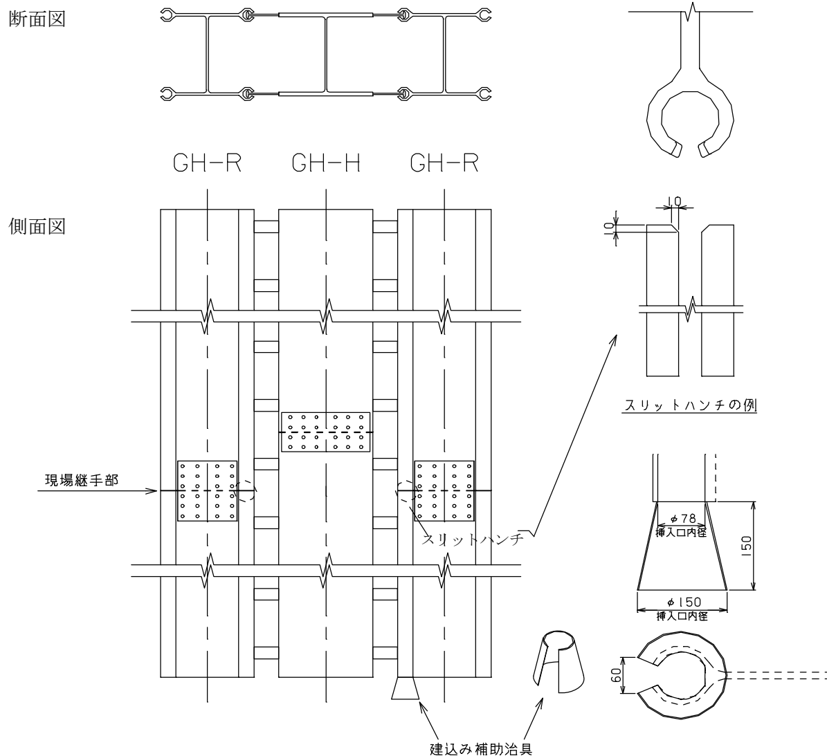
図－解 3.5.4 スリットハンチの加工例 (GH-R タイプ)
