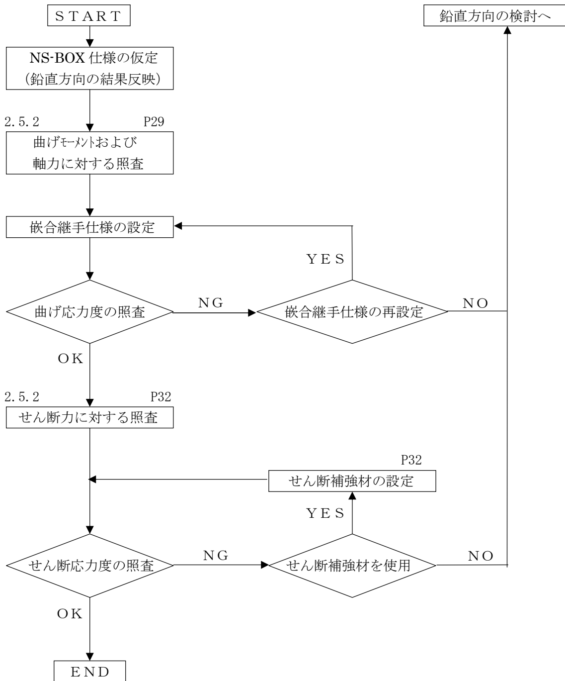
参考1 NS-BOX の設計フロー(水平方向)
