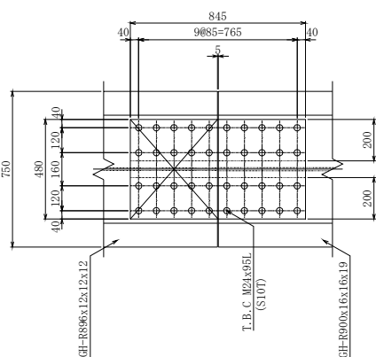
図一解 2.5.20 現場継手標準図
