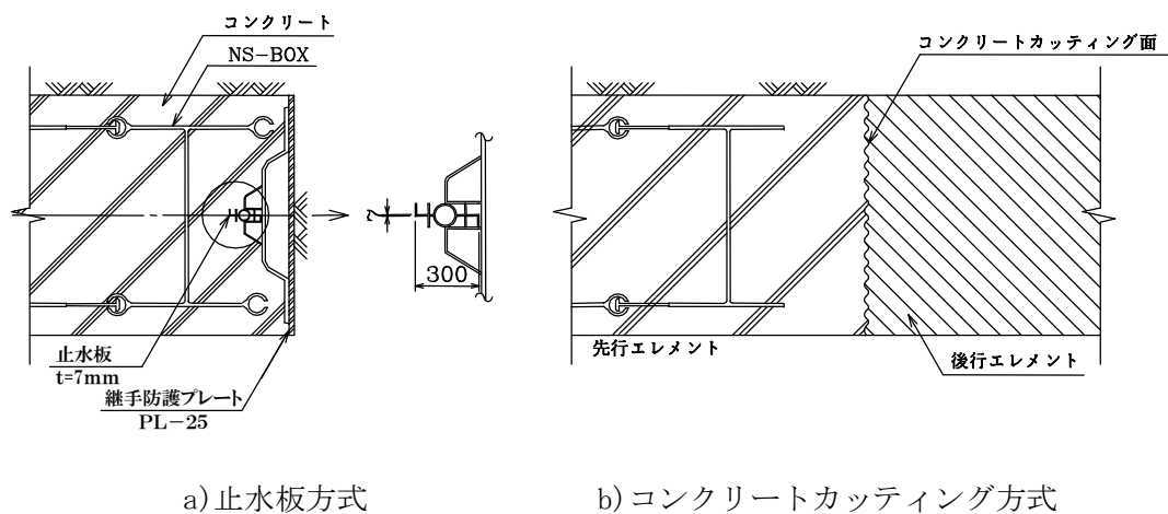
図一解 3. 6. 2 エレメント間継手の例
