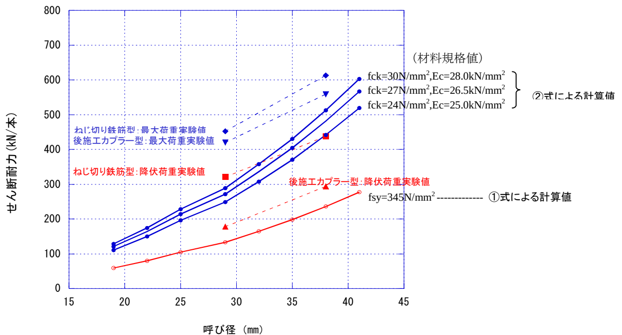
図一参 3.7 せん断耐力～鉄筋呼び径関係 (実験結果)
