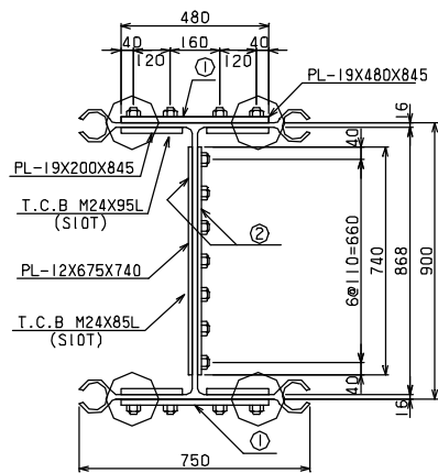
断面図
