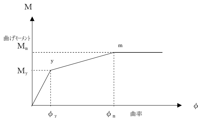
図一解 2.5.17 NS-BOX の曲げモーメントと曲率の関係
