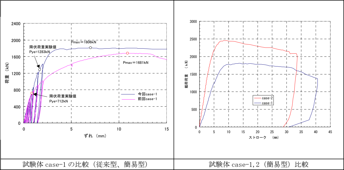
図一参 3. 3 耐力比較グラフ
