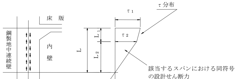
図一解2.5.26 該当するスパンにおける同符号の設計せん断力
