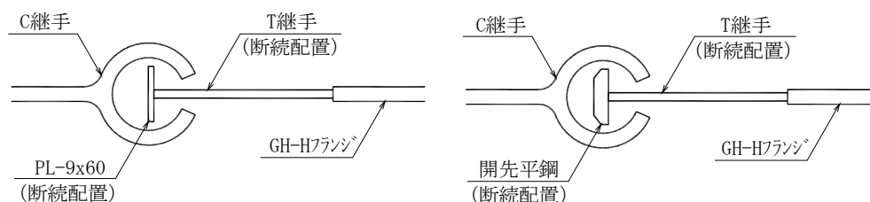
図-1.2.4 嵌合継手
