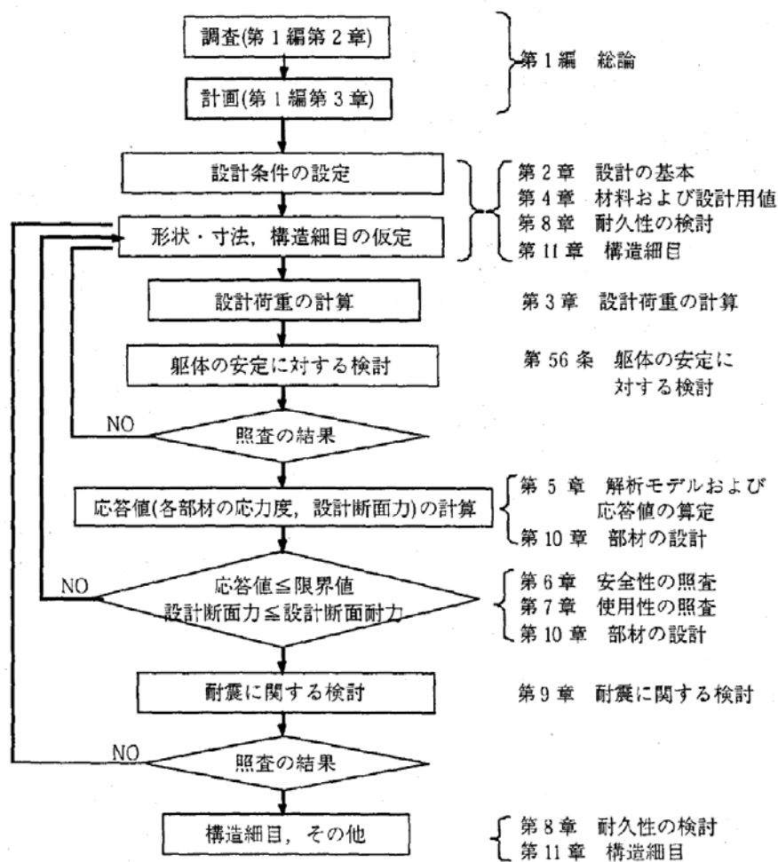
図一参 2.1 開削トンネルの設計フロー
