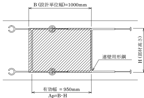
図一解 2.5.18 先端面積
