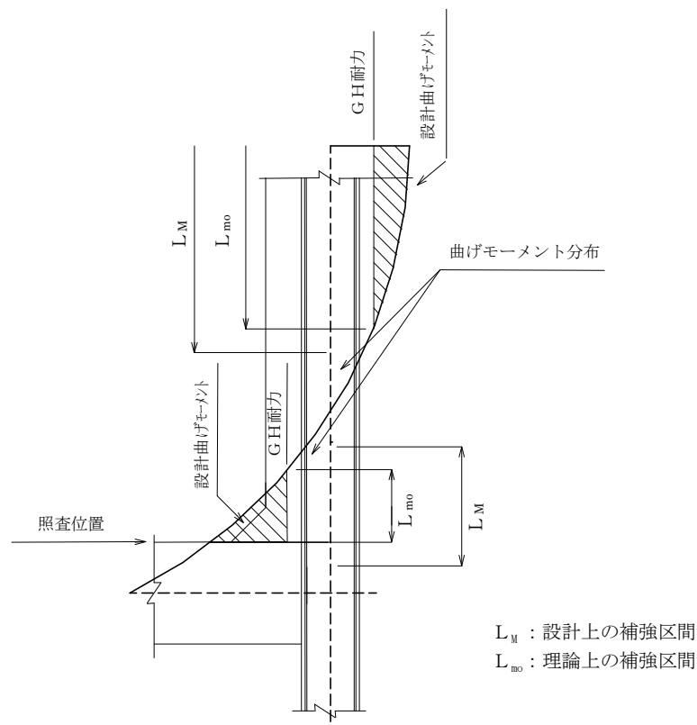
図一解 2.5.4 フランジ補強の範囲
