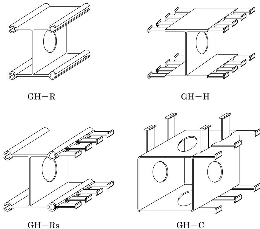
図－1. 2. 1 鋼製連壁部材
