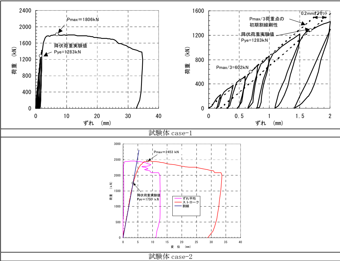
図一参 3.2 降伏荷重算定図
