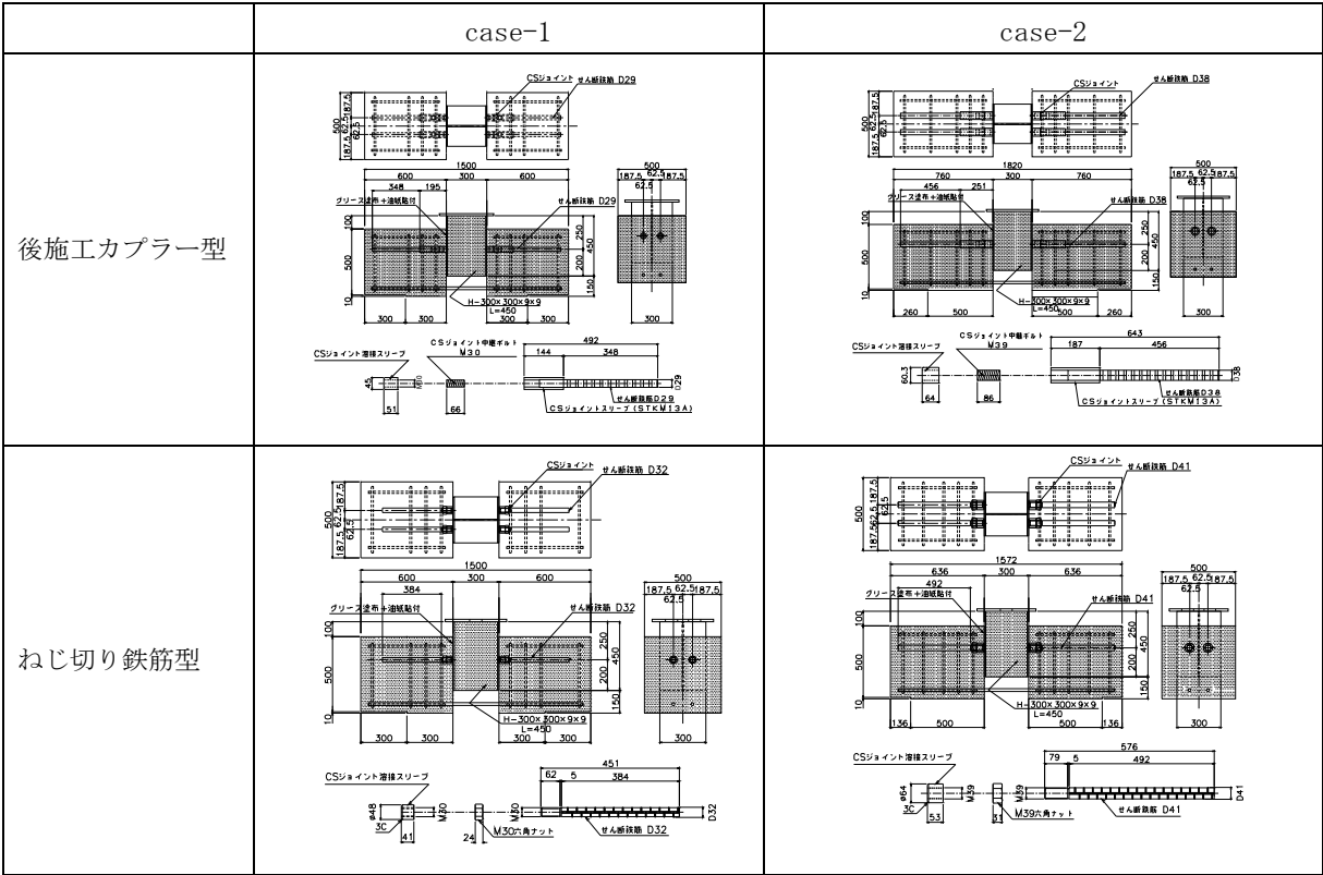
図一参 3.1 試験体・CSジョイント形状図
