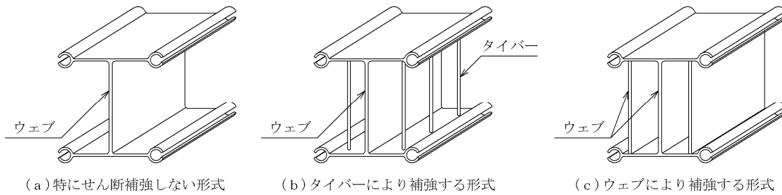
図一解 2.5.12 水平方向のせん断力に対する補強の形式
