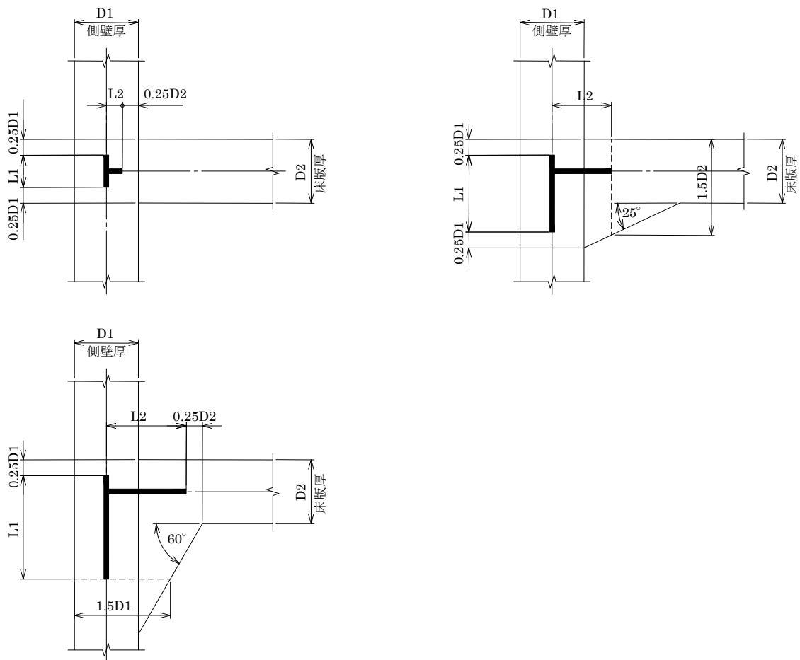
図－解 2.4.4 剛域の設定
