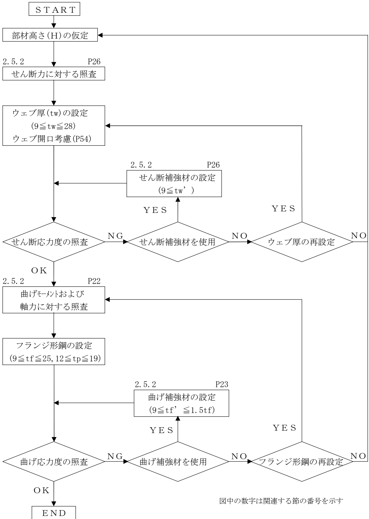
参考1 NS-BOX の設計フロー(鉛直方向)
